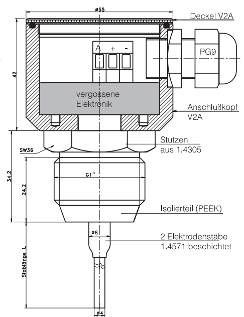
Maßzeichnung NVS-345.2w/...
