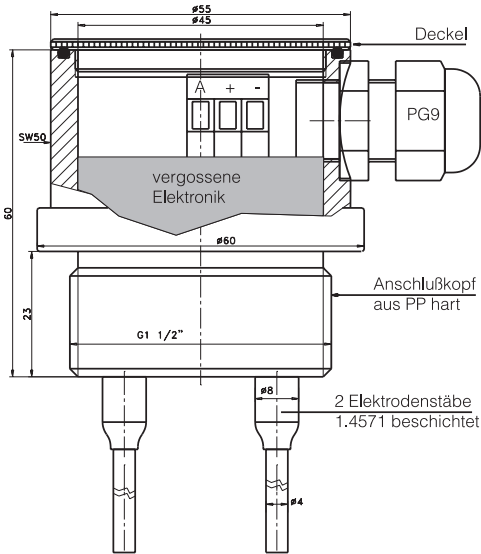
Maßzeichnung NVS-116.2w/...
