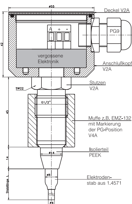
Maßzeichnung NVS-146.w/...
